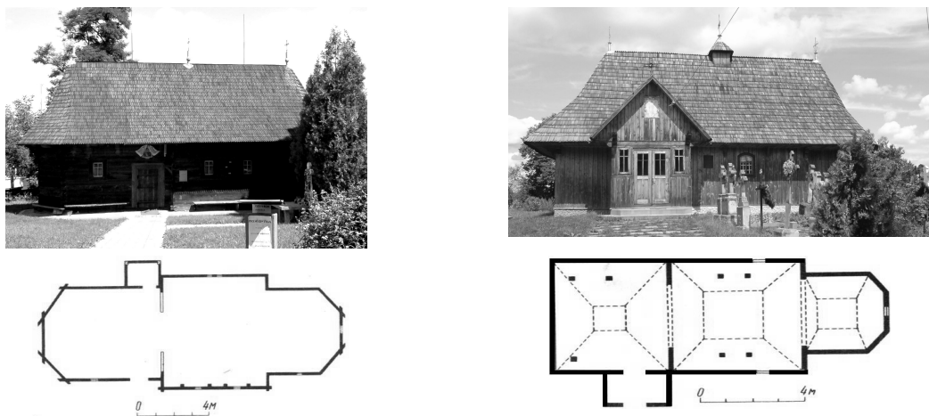
Рис. 5. Миколаївська церква, 1607 р.; Вознесенська церква, кінець XVII ст., м. Чернівці. Фото автора, 2008 р., плани [3].
