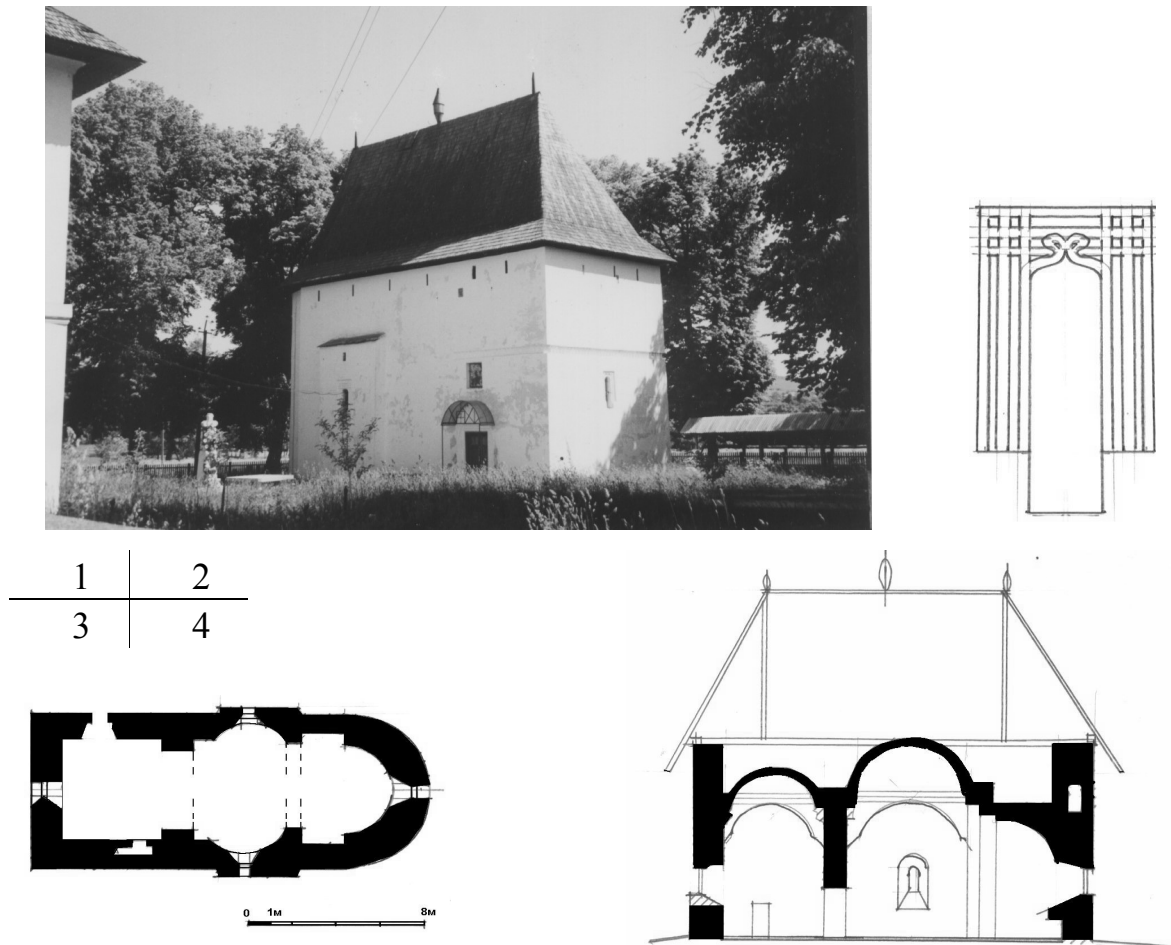
Рис. 4. Свято – Ільїнська церква у с. Топорівці Новоселицького району Чернівецької обл., 1560 рік. 1. Загальний вид фото автора, 2006 р.; 2. Кам'яний декор обрамлення вікна, рис. авт; 3. План; 4. Розріз (3,4- авторські, за матеріалами проекту реставраційних робіт Укрзахідпроектреставрація)
