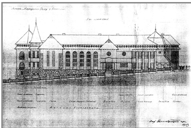
Начерк Народного Дому в Рогатині. Арх. Роман Грицай. 1923.
