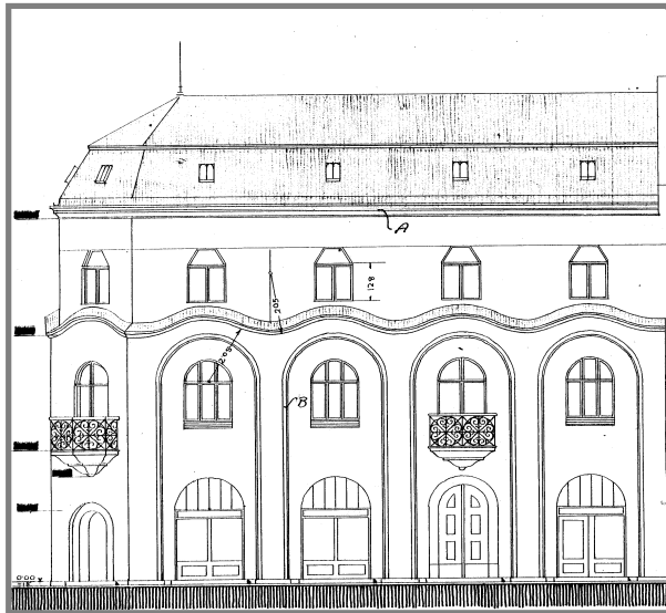
Дім Союзу Кооператив. Арх. Роман Грицай. 1926. Головний фасад.
