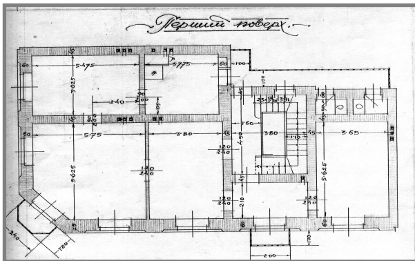
Дім Союзу Кооператив. Арх. Роман Грицай. 1926. План на відм. 4,42
